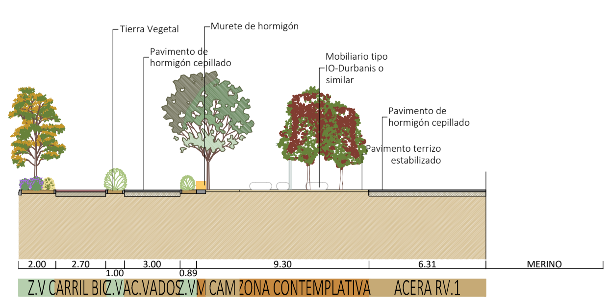
SECCIÓN RV 1.1 C-C' (E: 1/200)
