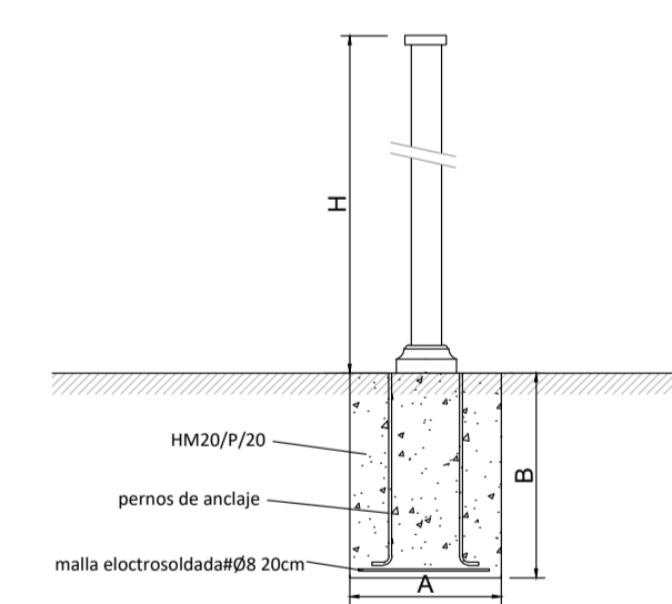
CIMENTACION
