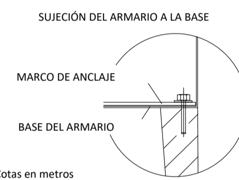
DETALLE C
