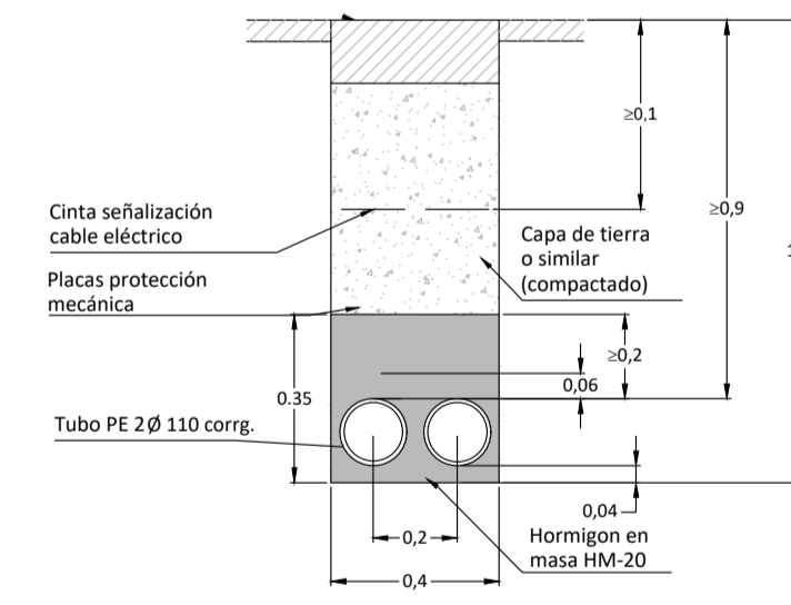
ZANJA CANALIZACION SEMAFOROS
