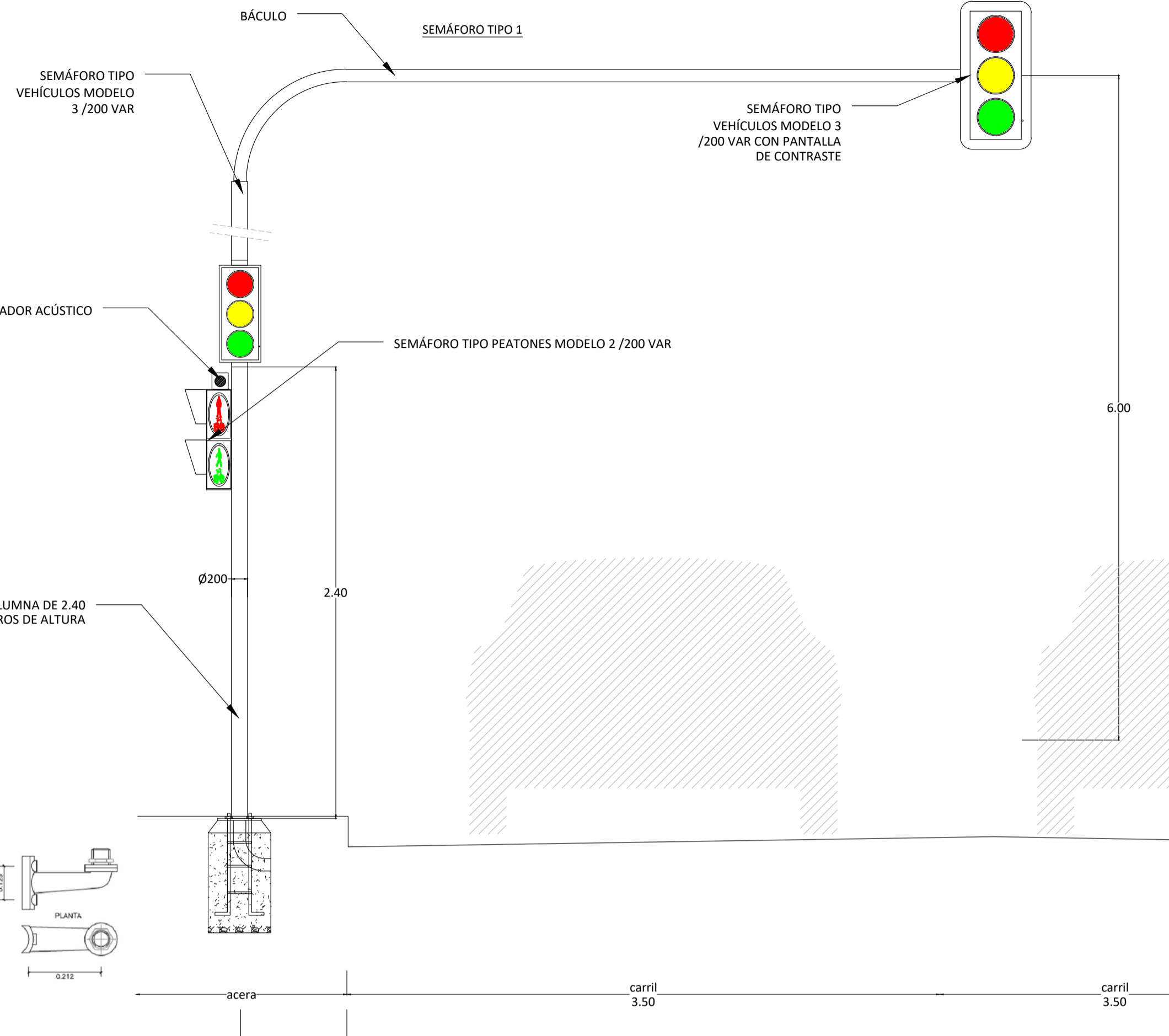
SEMÁFORO TIPO VEHICULOS MODELO 3 /200 VAR CON PANTALLA DE CONTRASTE
