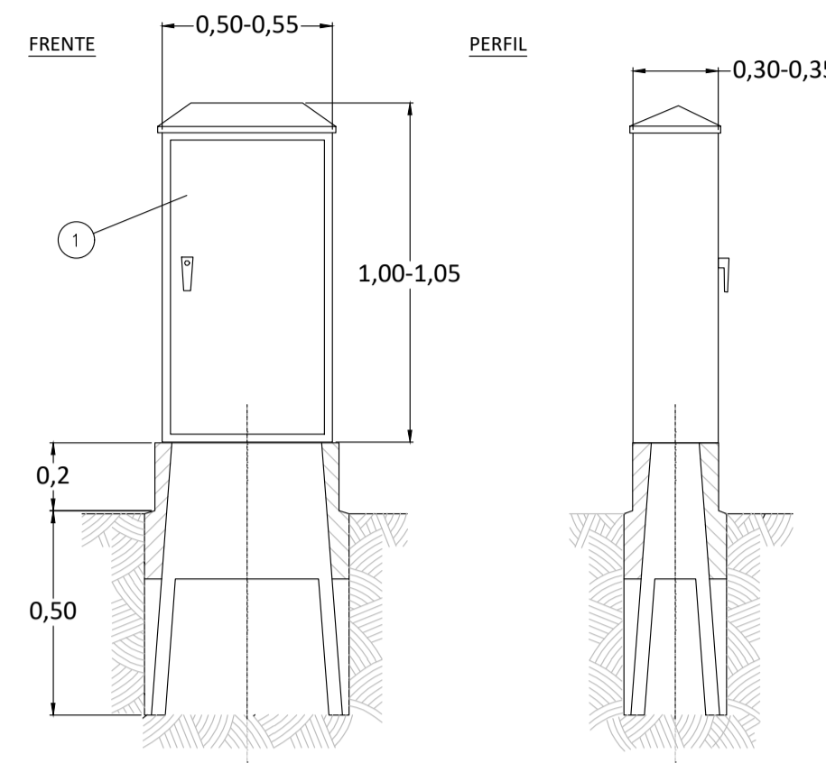
ARMARIO DE DISTRIBUCIÓN URBANA (ADU)
