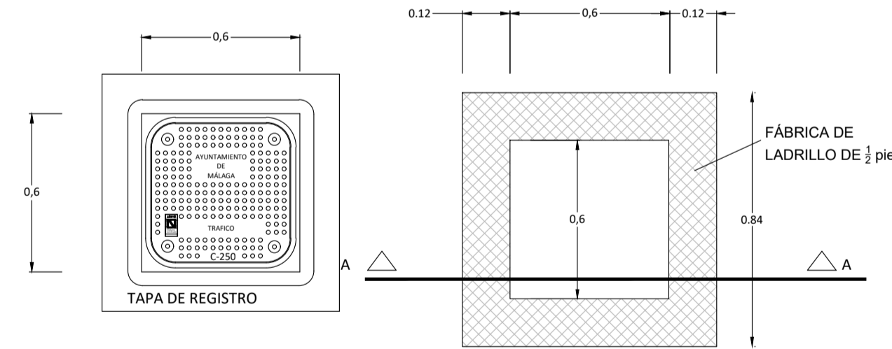
ARQUETA DE REGISTRO PARA SEMAFORIZACION DE 60x60 cm. CON TAPA DE FUNDICIÓN (C250). S/E COTAS EN m.
