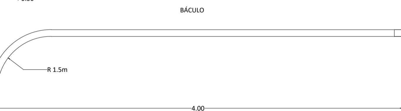
SEMÁFORO TIPO 2
