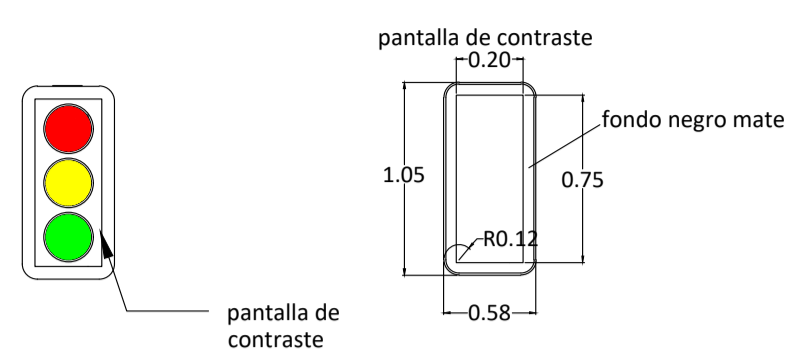
SEMÁFORO TIPO VEHICULOS MODELO 3 /200 VAR
