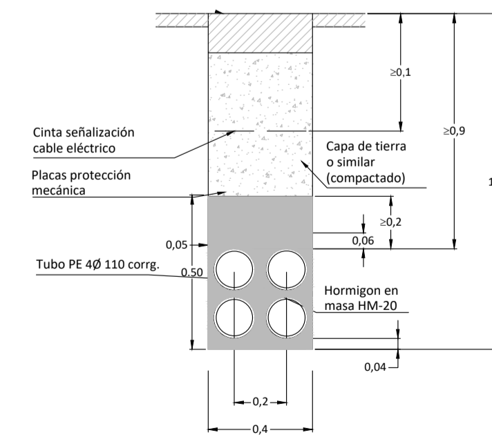
ZANJA CANALIZACION SEMAFOROS
