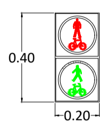
SEMÁFORO TIPO PEATONES/BICICLETAS MODELO 2 /200 VAR
