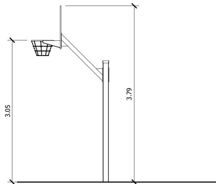
ALZADO 1/50
