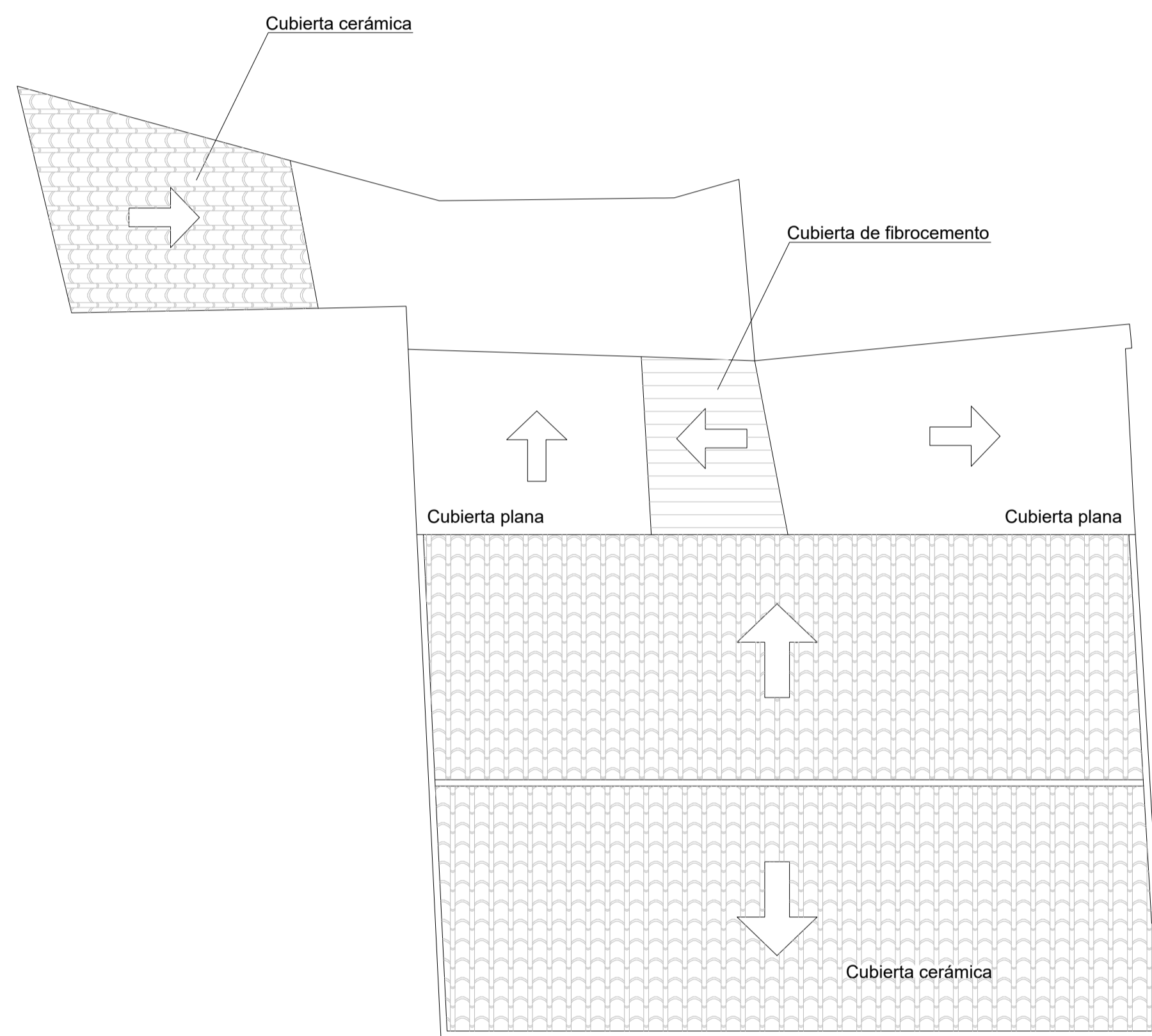
CUBIERTA
