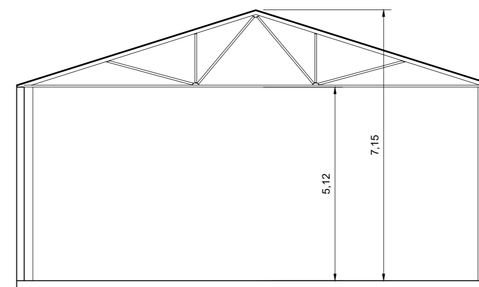
SECCIÓN A-A
