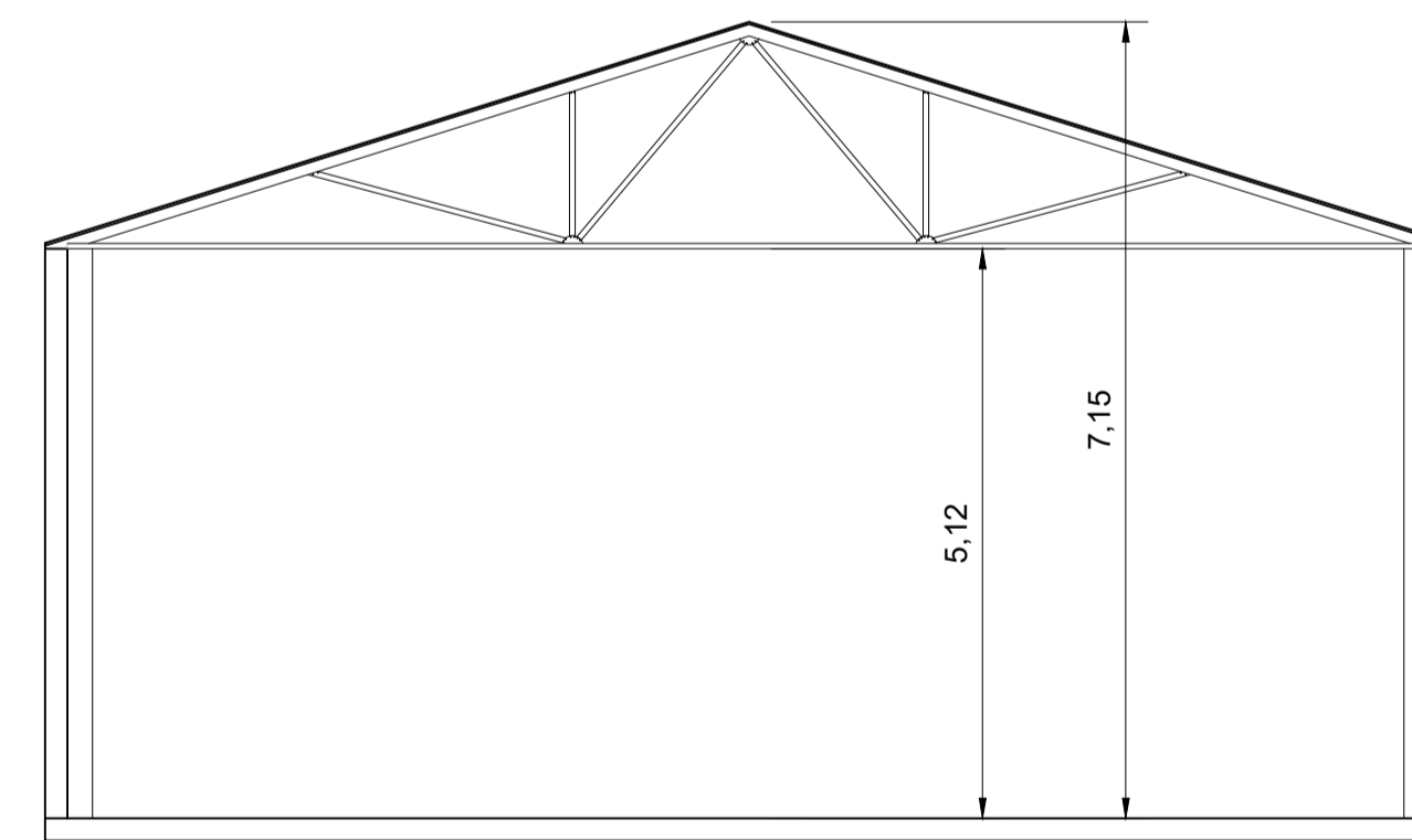
SECCIÓN A-A
